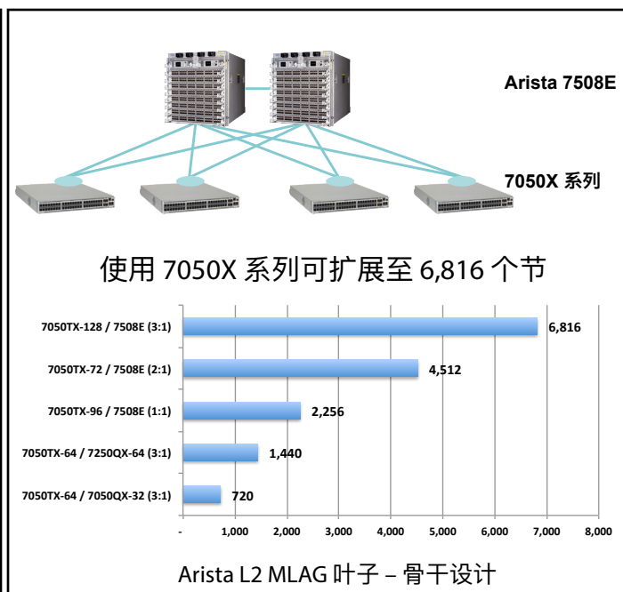
使用 Arista 叶子-骨干设计互连的 10GbE 节点数
