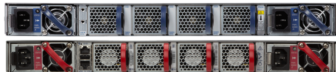
Arista 7050X 1RU 后视图：后端到前端气流型号 (蓝色) 前端到后端气流 (红色)
